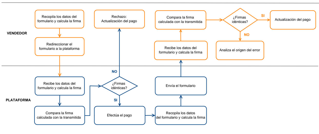
Figura 8: Diagrama mecanismo de seguridad
